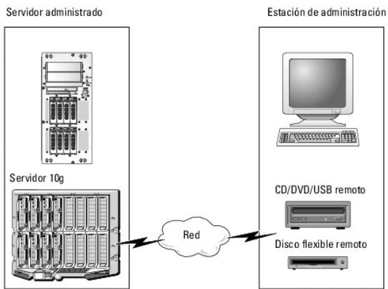
Figura 8-1. Arquitectura general de medios virtuales
